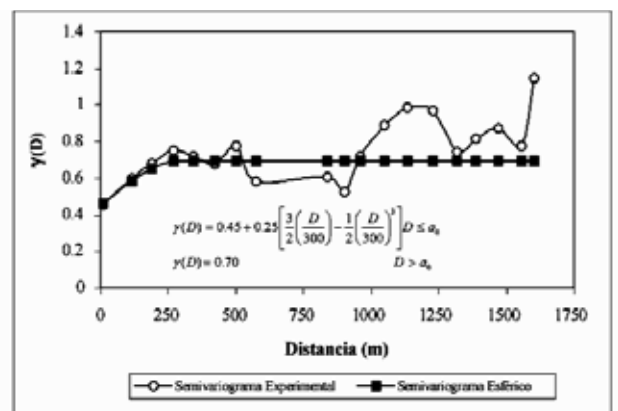
Figura 5 y 6. Semivariograma para \text{Ln} Sorptividad (superficie) con en la serie de suelos Comelles y Semivariograma para \text{Ln}K_s (horizonte Ap) en la serie de suelos Seana
