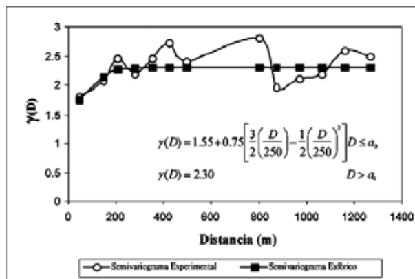
Figura 3 y 4. Semivariograma para \text{Ln}K_s (horizonte Ap) en la serie de suelos Comelles y Semivariograma para \text{Ln}K_s (superficie) con en la serie de suelos Comelles
