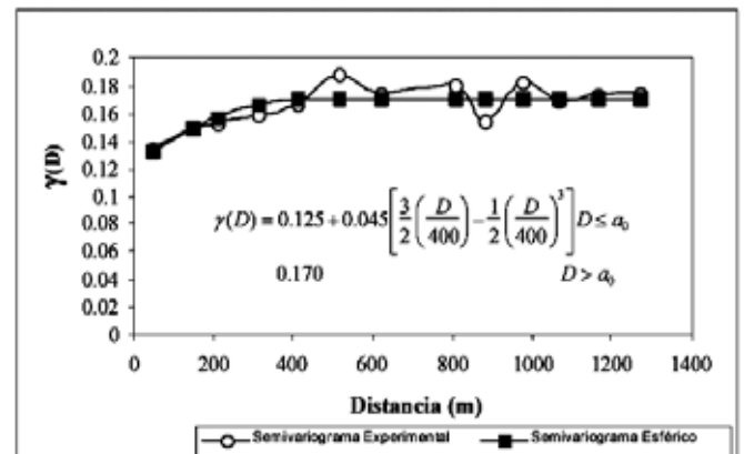
Figura 3 y 4. Semivariograma para \text{Ln}K_s (horizonte Ap) en la serie de suelos Comelles y Semivariograma para \text{Ln}K_s (superficie) con en la serie de suelos Comelles
