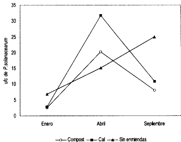
Figura 2. Comportamiento de las poblaciones de P. solanacearum en parcelas con enmiendas de compost (40 t.ha -1 ), cal dolomítica (5 t.ha -1 ) y en parcelas sin enmiendas. Estación Experimental La Montaña, Turrialba, Costa Rica. 1999.
